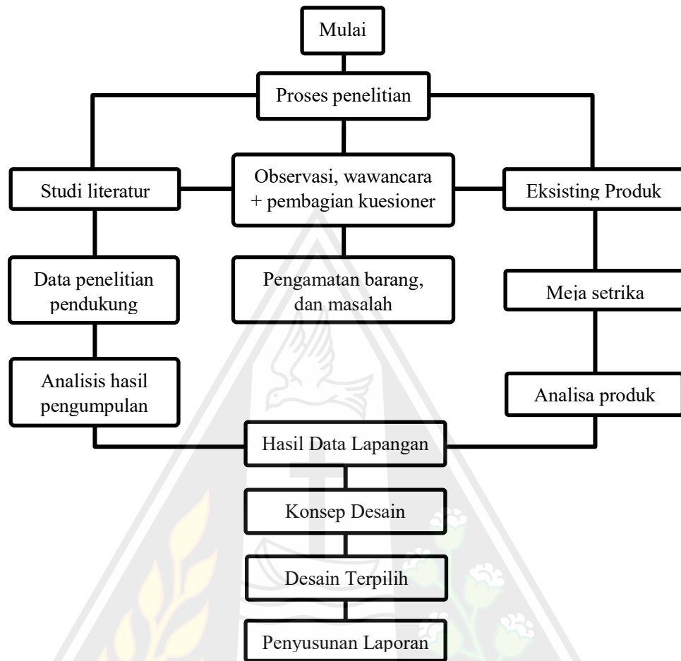
Diagram 1.1 Kerangka Berpikir
